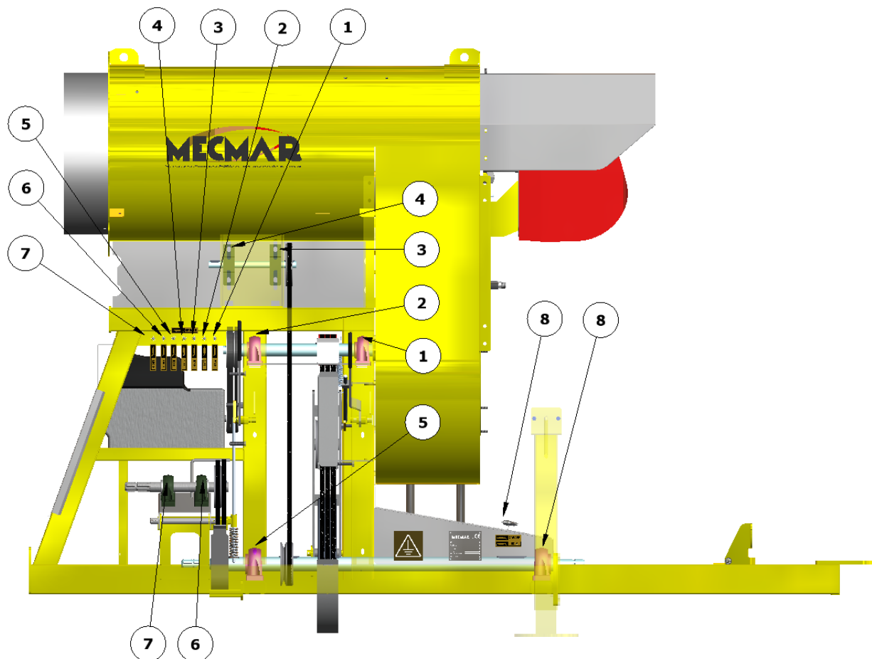
СРТ: ОСНОВНЫЕ ТОЧКИ СМАЗКИ ПРИ ПРИВОДЕ ОТ ВОМ – MAIN GREASING POINTS ON PTO HEAD
