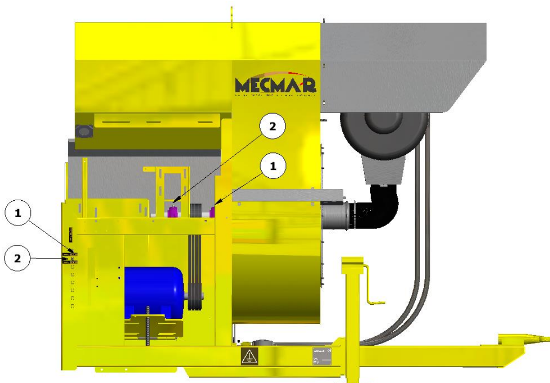
STR FSN D: ОСНОВНЫЕ ТОЧКИ СМАЗКИ ПРИВОД ОТ 1-го ЭЛЕКТРОДВИГАТЕЛЯ - MAIN GREASING POINTS ON 1 M.E. HEAD
