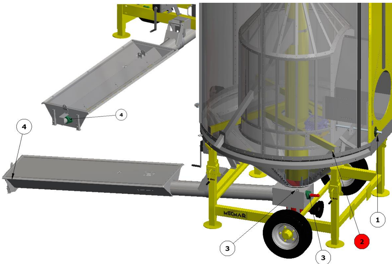
СРТ: ОСНОВНЫЕ ТОЧКИ СМАЗКИ ЦИЛИНДРА – MAIN GREASING POINTS ON CYLINDER
