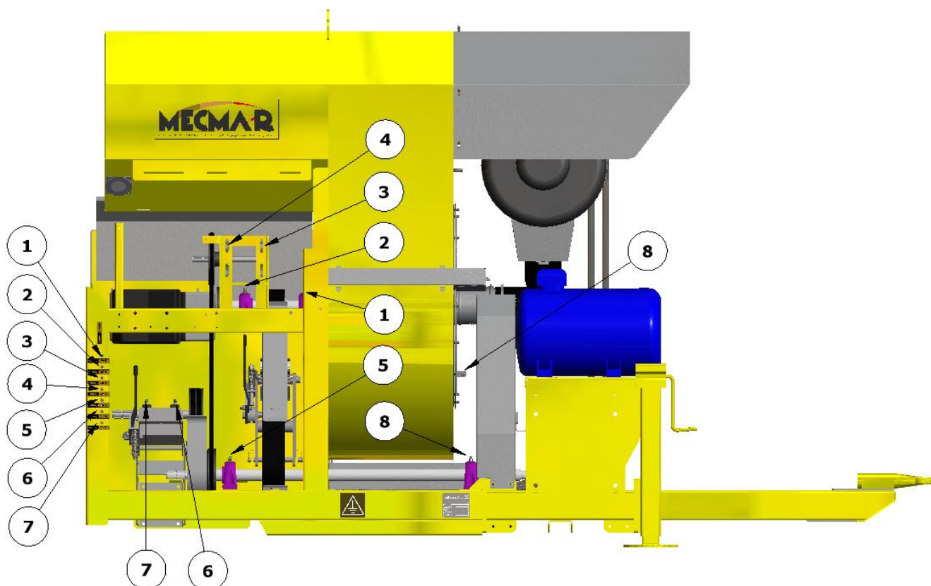
STR FSN D: ОСНОВНЫЕ ТОЧКИ СМАЗКИ ПРИВОДА ОТ ВОМ + 1 ЭЛЕКТРОДВИГАТЕЛЬ – MAIN GREASING POINTS ON PTO +1 M.E. HEAD
