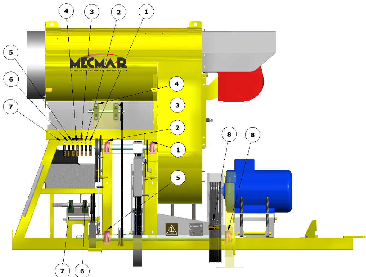
СРТ: – ОСНОВНЫЕ ТОЧКИ СМАЗКИ ПРИ ПРИВОДЕ ОТ ВОМ + ЭЛЕКТРОДВИГАТЕЛЬ MAIN GREASING POINTS ON PTO + 1 M.E. HEAD
