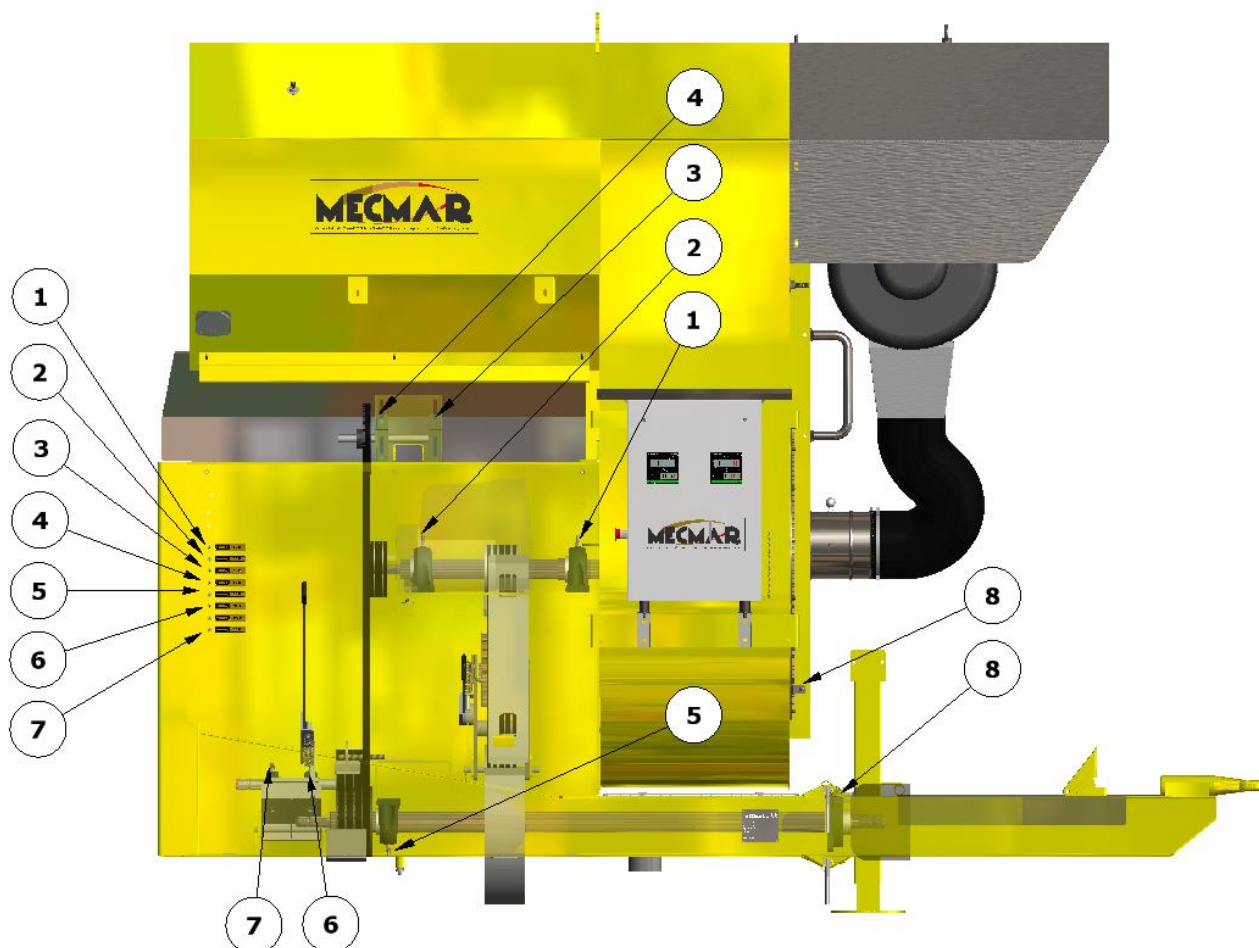
SSI: ОСНОВНЫЕ ТОЧКИ СМАЗКИ ПРИ ПРИВОДЕ ОТ ВОМ– MAIN GREASING POINTS ON PTO HEAD
