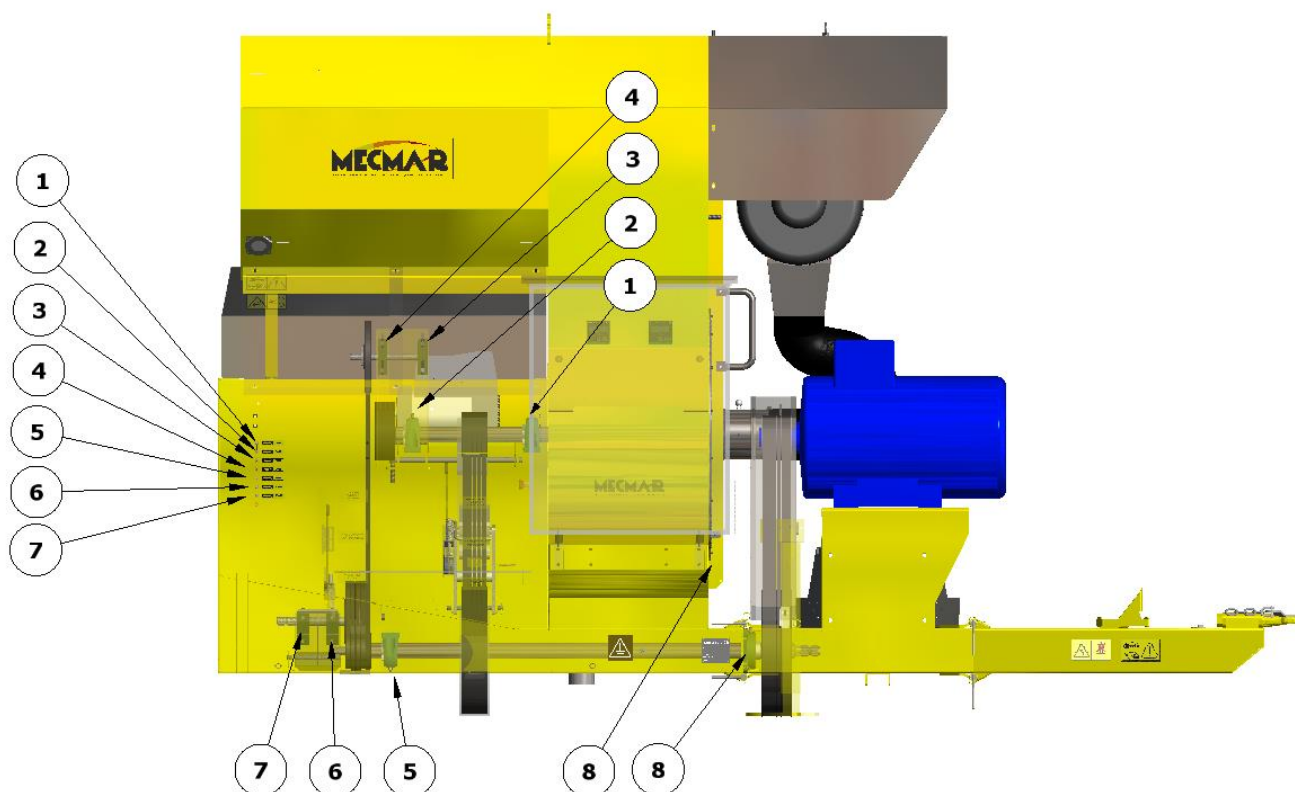
S : ОСНОВНЫЕ ТОЧКИ СМАЗКИ ПРИ ПРИВОДЕ ОТ ВОМ + 1 ЭЛЕКТРОДВИГАТЕЛЬ – MAIN GREASING POINTS ON PTO +1 M.E. HEAD
