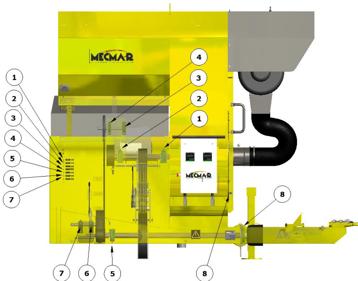
S: ОСНОВНЫЕ ТОЧКИ СМАЗКИ ПРИ ПРИВОДЕ ОТ ВОМ – MAIN GREASING POINTS ON PTO HEAD
