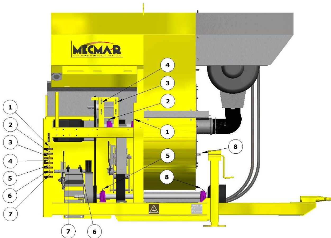
STR FSN D: ОСНОВНЫЕ ТОЧКИ СМАЗКИ ПРИВОДА ВОМ– MAIN GREASING POINTS ON PTO HEAD
