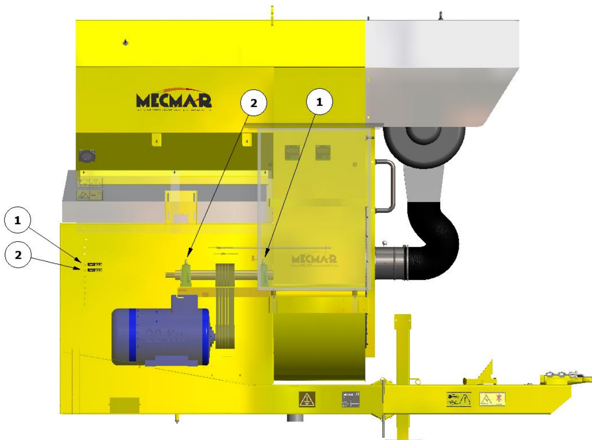
SSI: ОСНОВНЫЕ ТОЧКИ СМАЗКИ ПРИВОД ОТ 1-го ЭЛЕКТРОДВИГАТЕЛЯ – MAIN GREASING POINTS ON 1 M.E. HEAD
